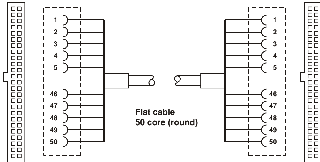
Wiring
